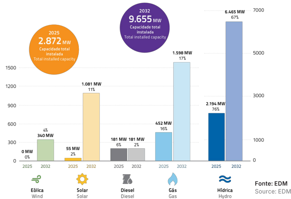
Capacidade instalada em 2025 e previsão 2032 Installed Capacity in 2025 and forecast 2032
