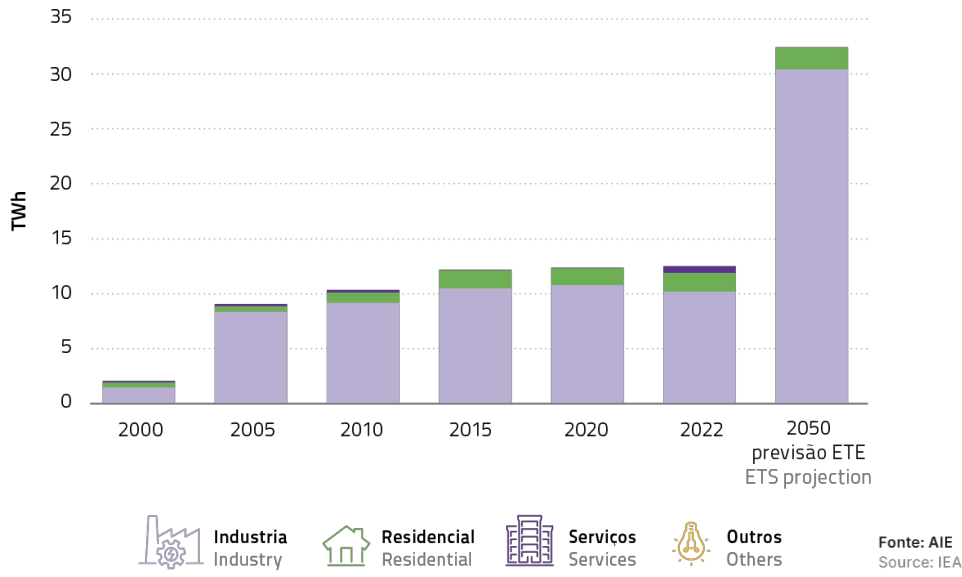
Evolução do consumo total de electricidade por sector Electricity total consumption by sector
