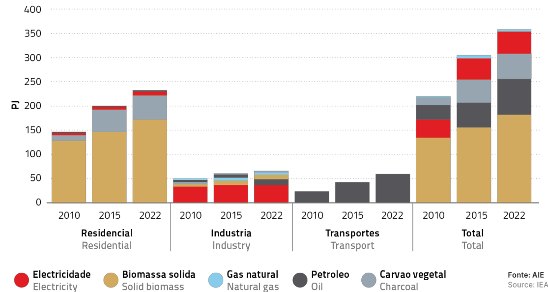
Consumo final total de energia, por combustível, nos sectores de utilização final Total final energy consumption by fuel in end-use sectors
