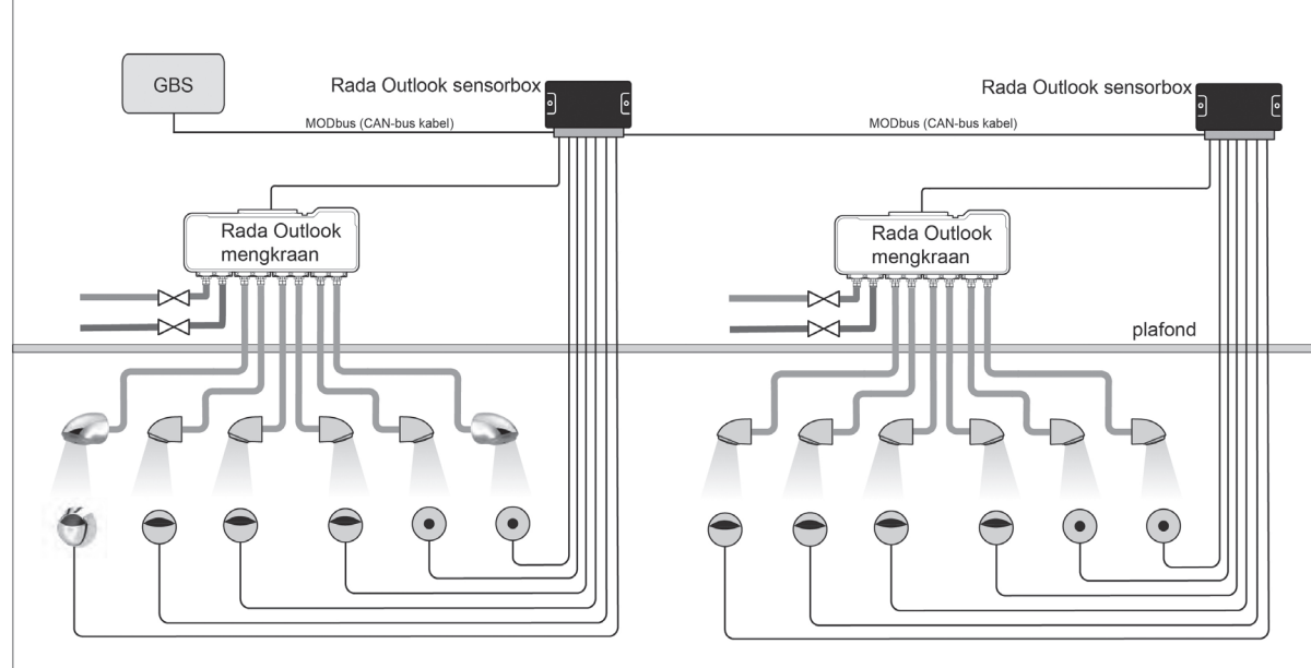
Meerdere Rada Outlook digitale mengkranen gekoppeld aan een GBS (MODbus)
